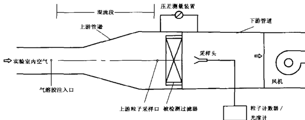
图 A.1 扫描检漏法检测示意图
